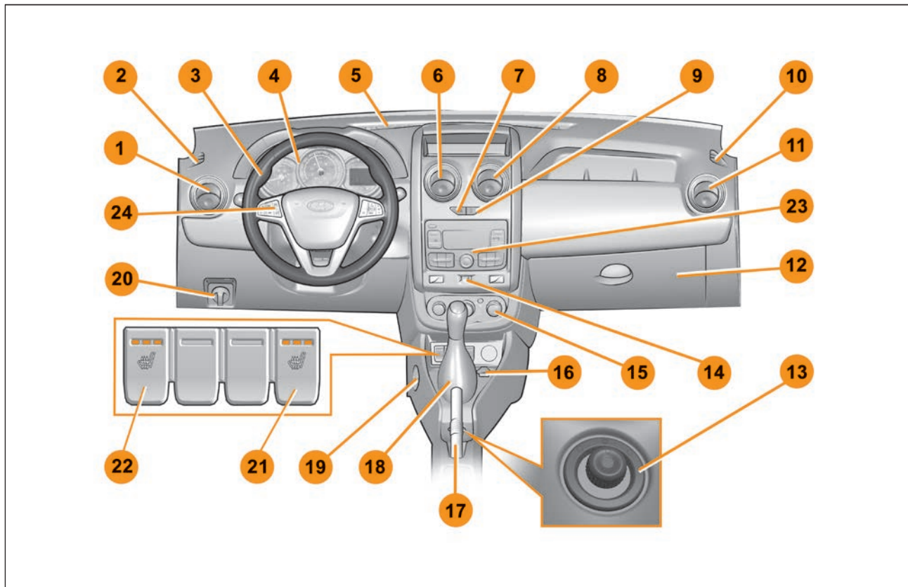
Рис. 3.1.2. Панель приборов в исполнении «Норма» (в варианном исполнении)
