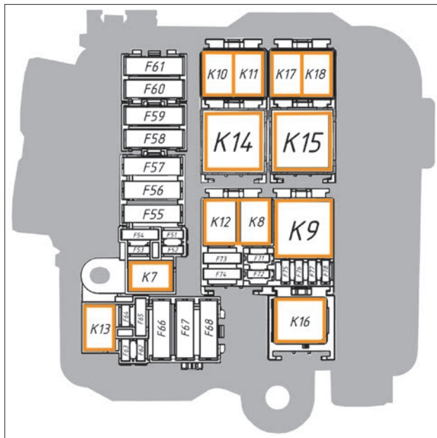
Рис. 8.4.2. Схема расположения предохранителей и реле в монтажном блоке моторного отсека (в варианном исполнении)
