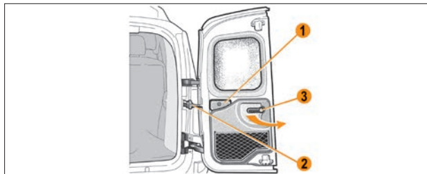
Рис. 1.4.7. Открытие меньшей двери багажного отделения
