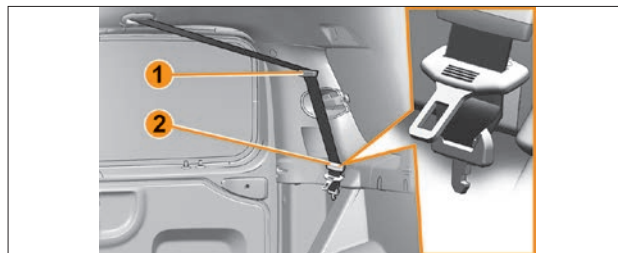
Рис. 2.5.7б. Фиксация среднего ремня безопасности (в варианном исполнении)
