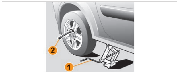
Рис. 6.9.3. Снятие колеса
